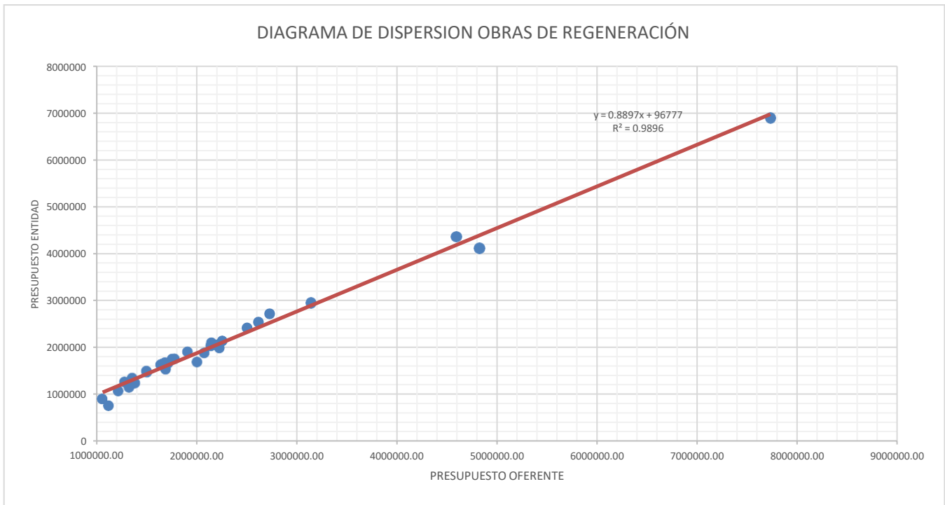
Ilustración 12: Diagrama de dispersión obras de regeneración Fuente: Autor
