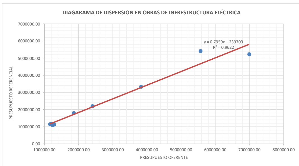
Ilustración 17: Diagrama de dispersión en obras de infraestructura eléctrica Fuente: Autor
