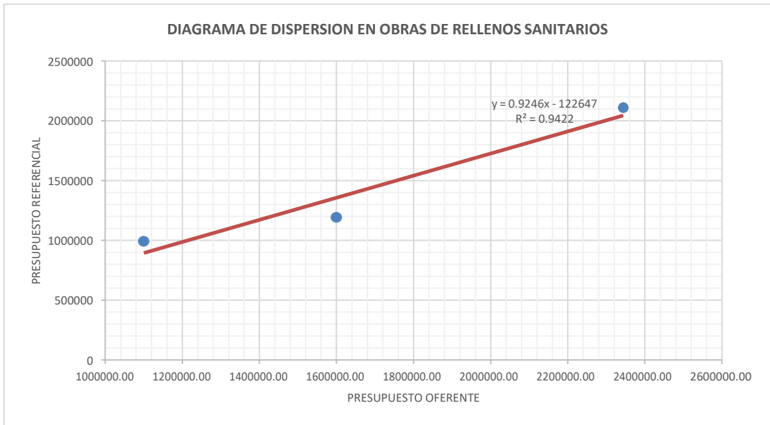
Ilustración 20: Diagrama de dispersión en obras de rellenos sanitarios Fuente: Autor
