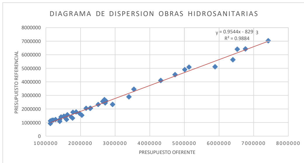
Ilustración 8: Diagrama de dispersión obras hidráulicas
