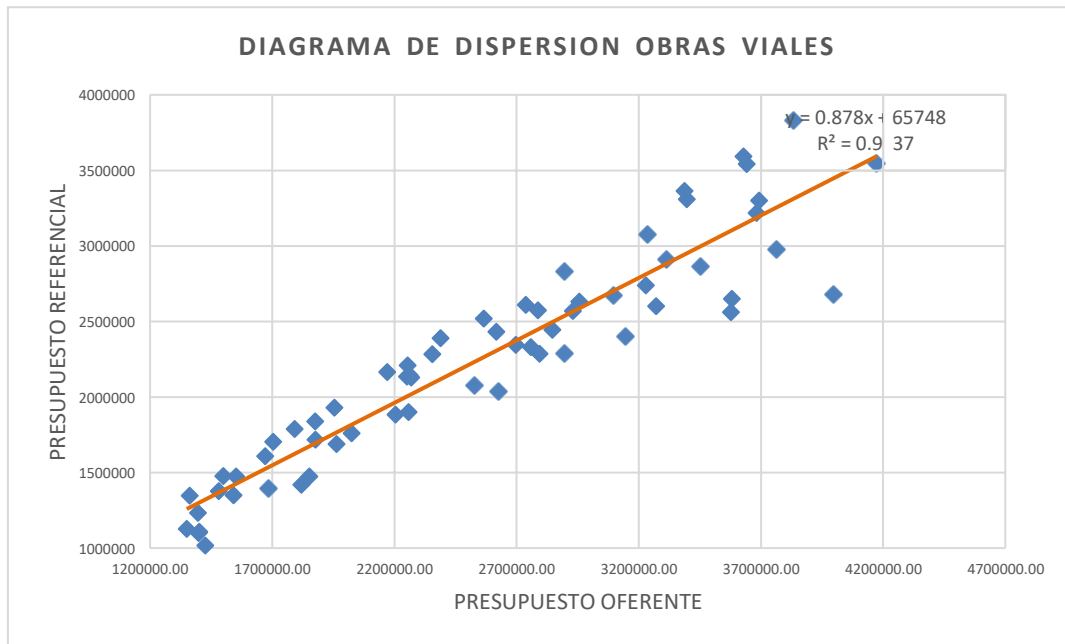
Ilustración 7: Diagrama de dispersión de obras viales Fuente: Autor
