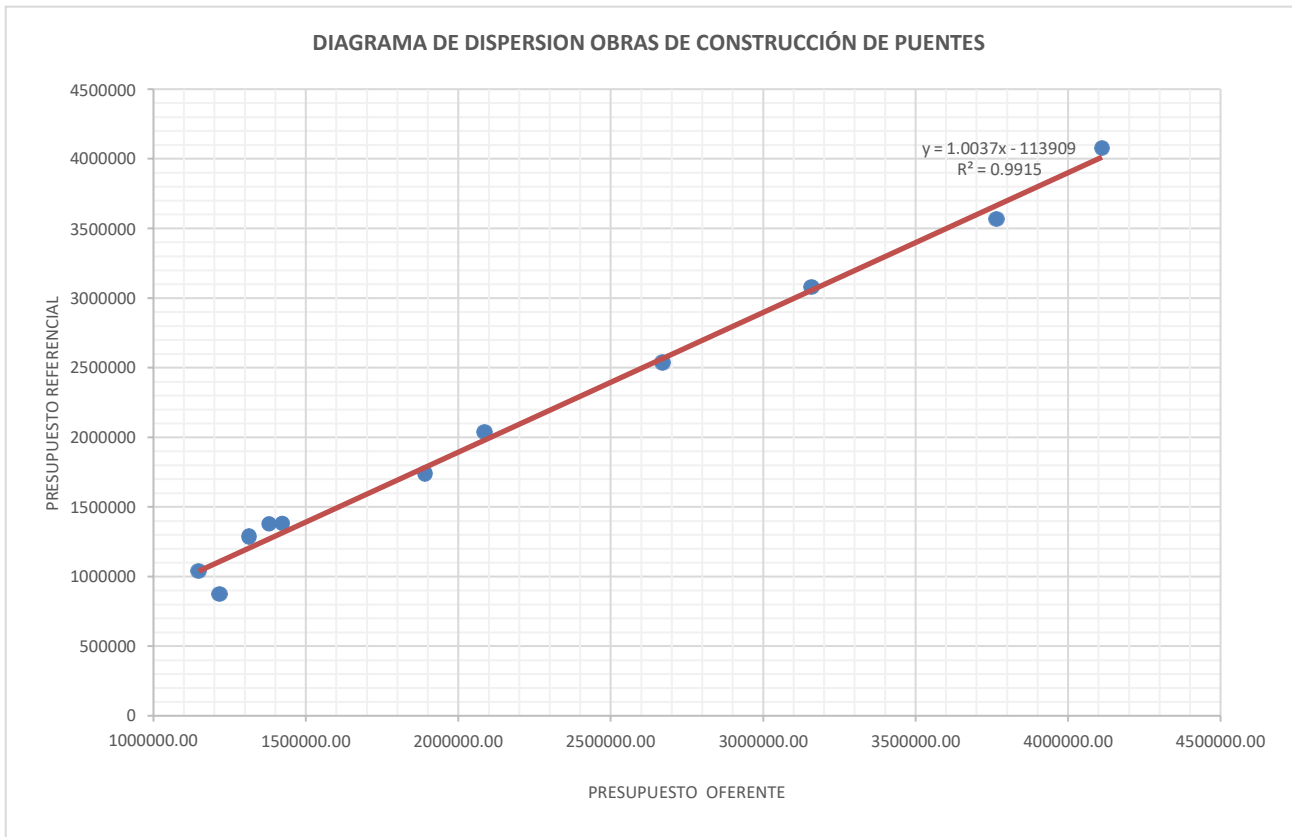
Ilustración 16: Diagrama de dispersión en obras de puentes Fuente: Autor
