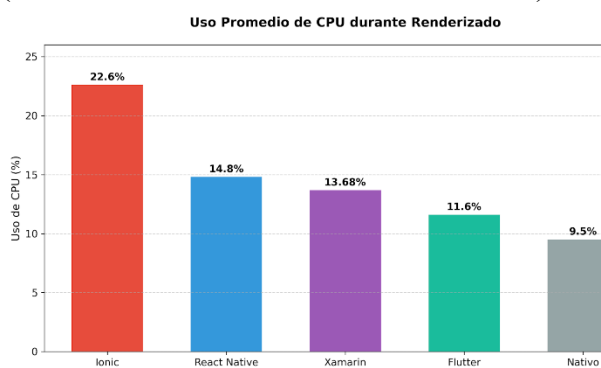
Figura 3: Consumo promedio de CPU durante tareas de renderizado gráfico. Nota. Datos procesados a partir de las métricas de rendimiento de (Kodithuwak & Pacillo, 2025).
