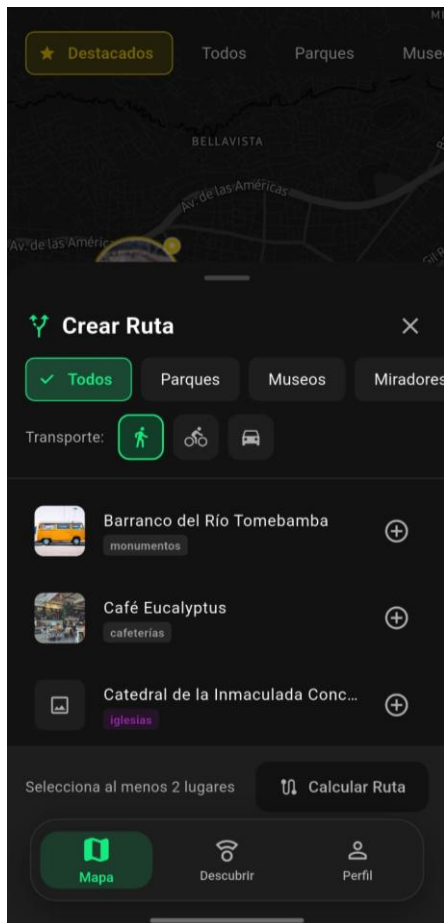
Figura 8: Interfaz de planificación de rutas.
