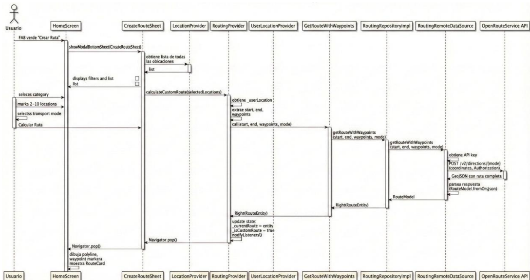
Figura 6: Diagrama de flujo lógico para la generación de ruta.
