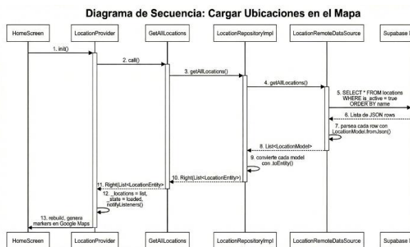
Figura 5: Diagrama de secuencia de la carga de datos geoespaciales.
