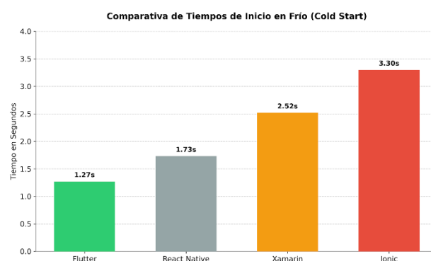
Figura 2: Comparativa de tiempos promedio de inicio en frío (Cold Start) entre frameworks multiplataforma. Nota. Datos adaptados de (Kodithuwak & Pacillo, 2025).
