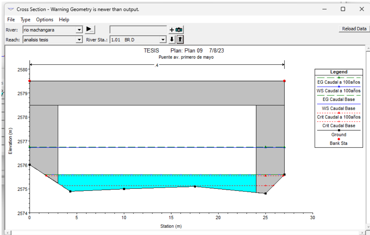
Ilustración 28 Análisis de caudales proyectados
