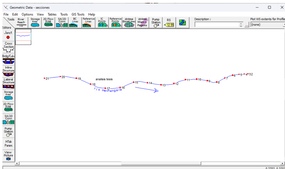
Ilustración 7 Datos de secciones en el programa de análisis de crecidas
