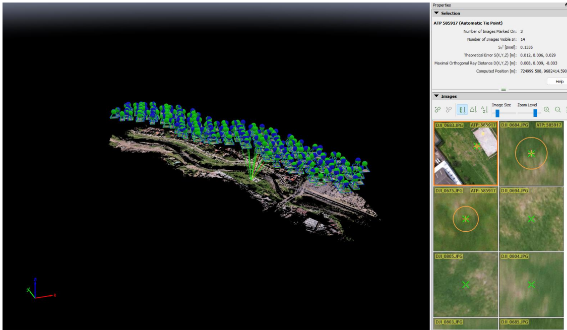
Ilustración 21 Creación de nube de puntos para topografía
