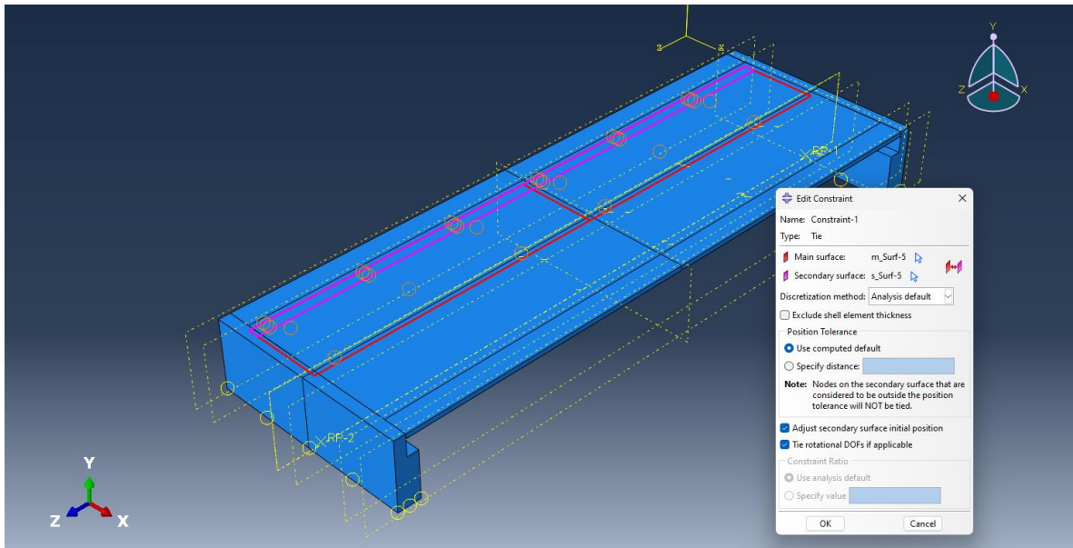
Ilustración 33 Asignación de interacciones entre elementos
