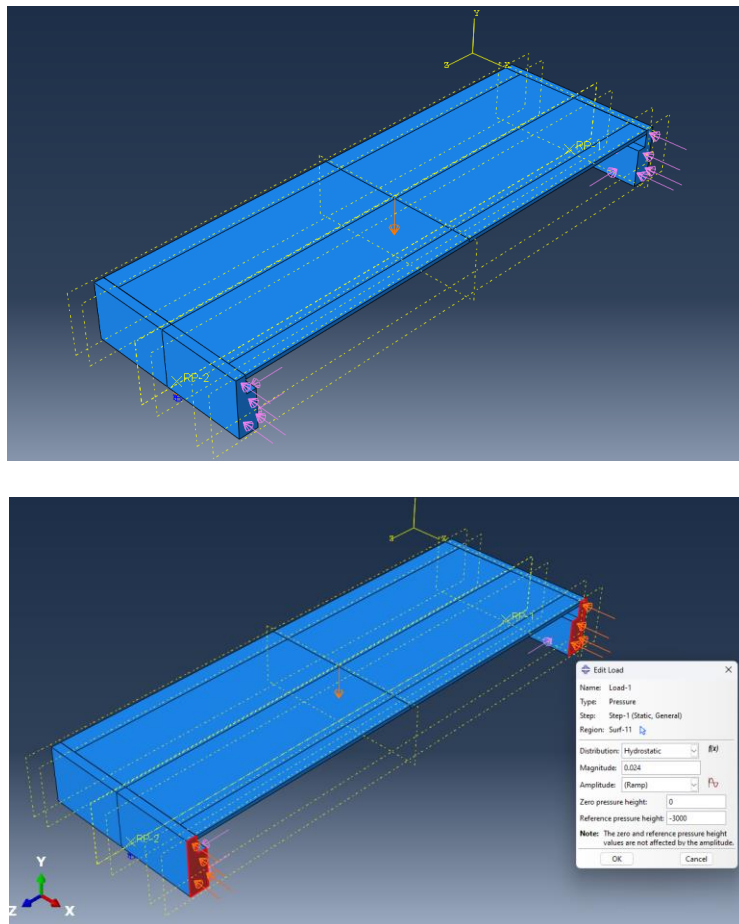
Ilustración 13 Cargas dinámicas insertadas
