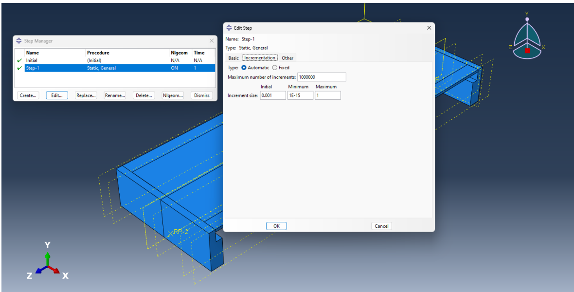
Ilustración 32 Creación del caso de carga
