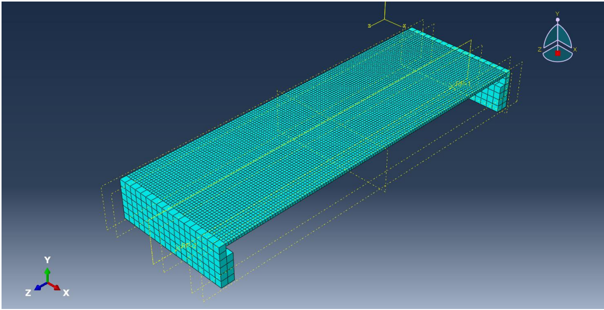
Ilustración 35 Mallado del modelo
