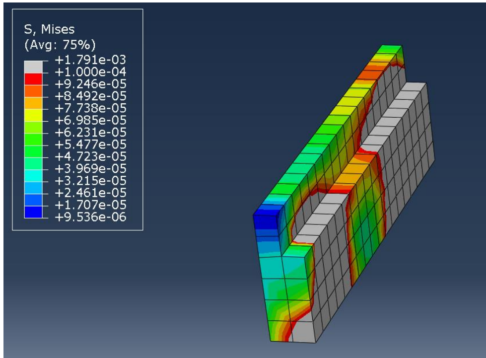
Ilustración 14 Modelo del estribo con cargas laterales del agua
