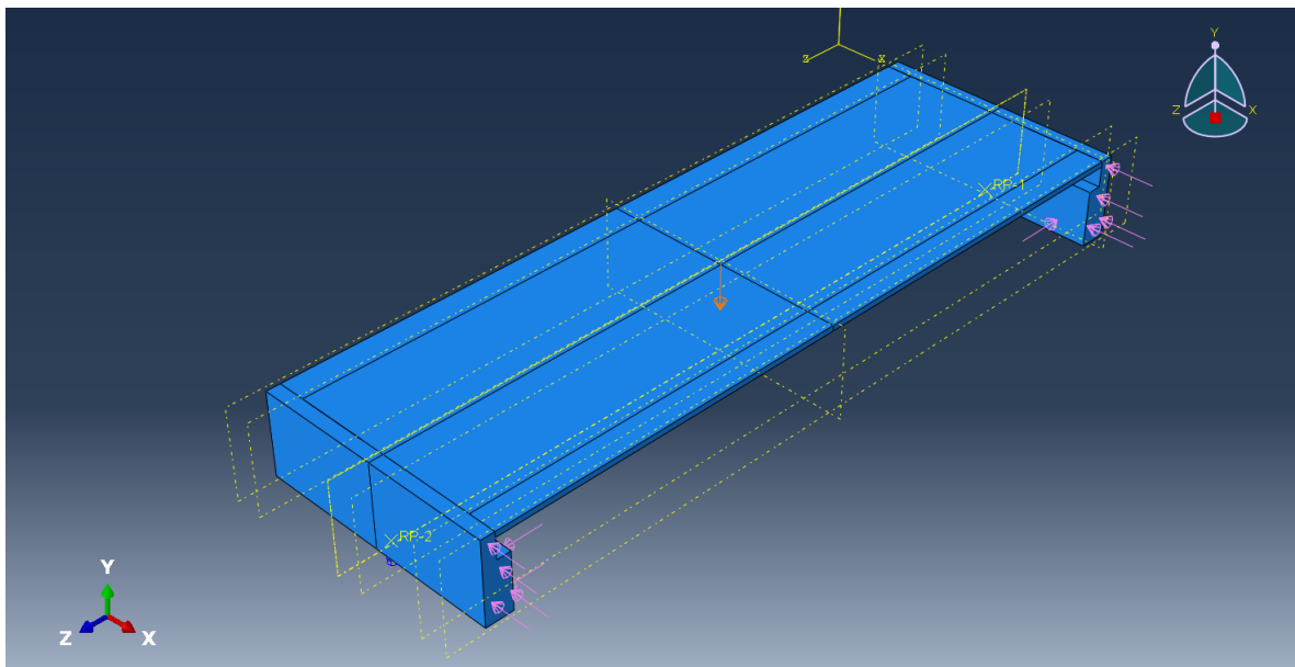
Ilustración 34 Asignación de cargas al elemento
