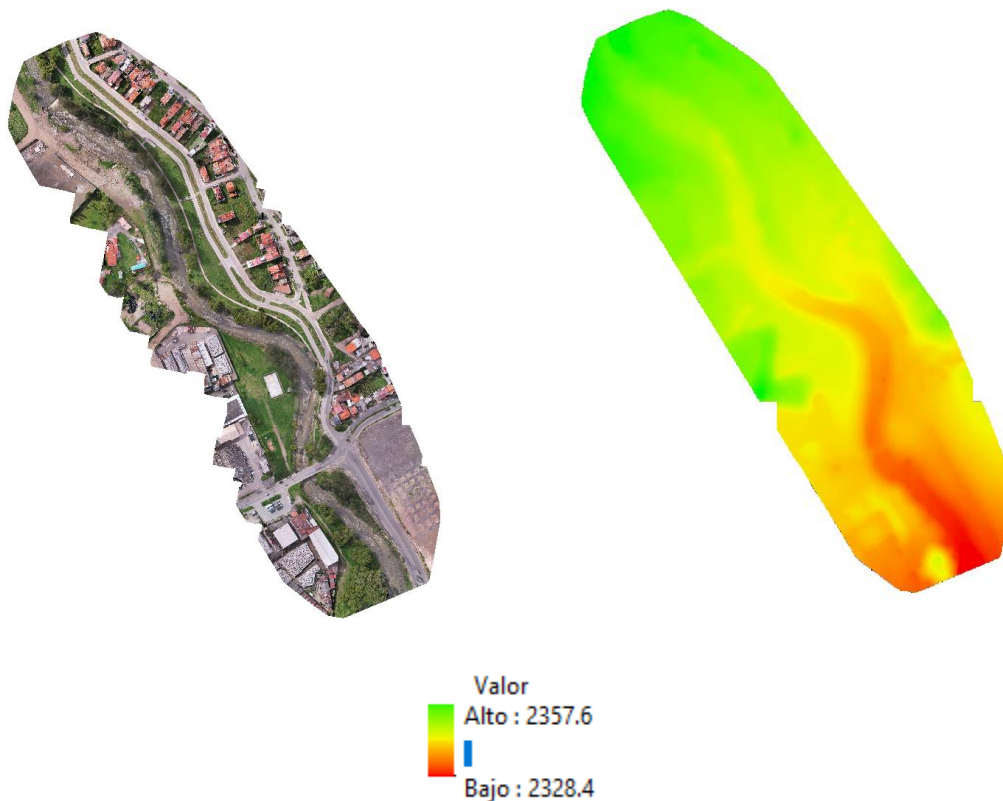
Ilustración 9 MDT del río
