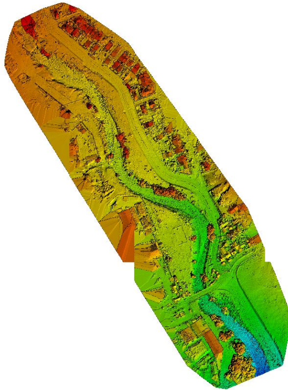
Ilustración 24 DSM
