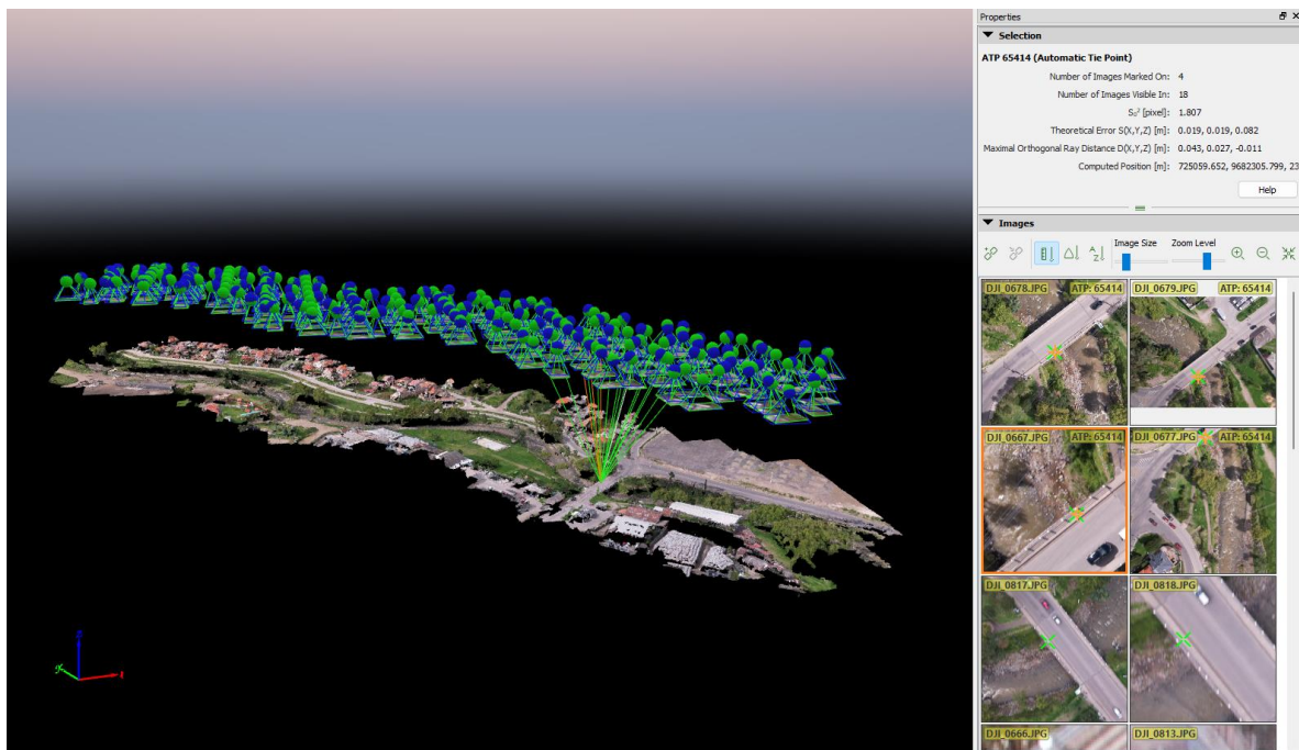
Ilustración 3 Análisis de fotogrametría mediante software de fotogrametría
