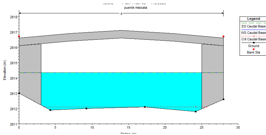
Ilustración 11 puente con calado de 3m
