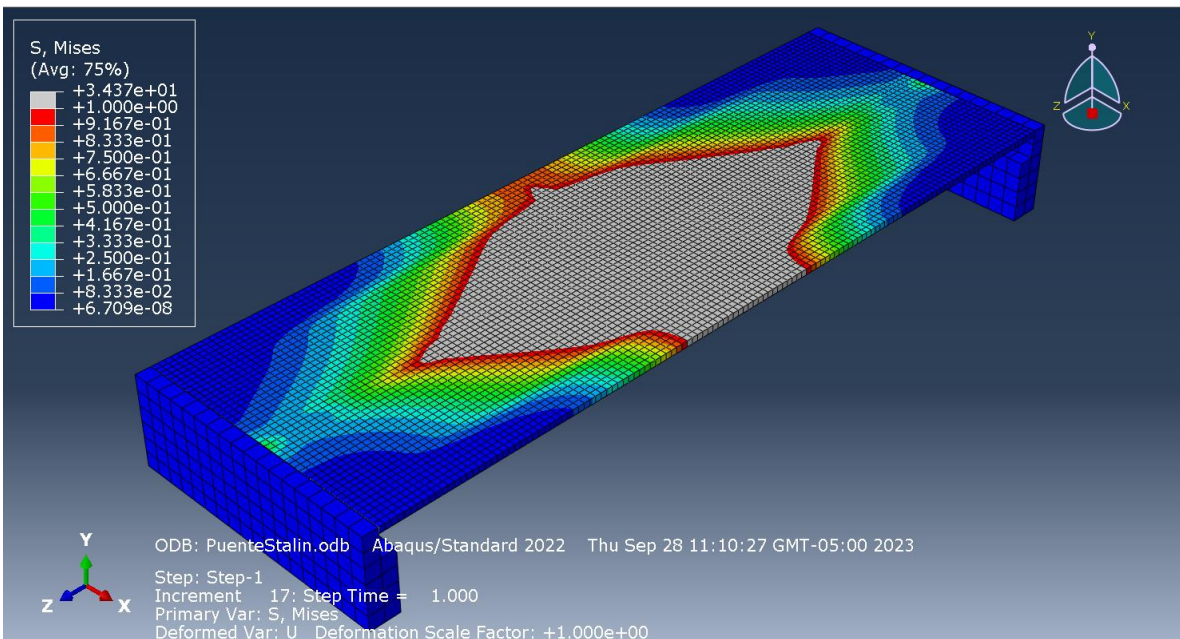
Ilustración 36 Análisis de esfuerzos en modelo FEM
