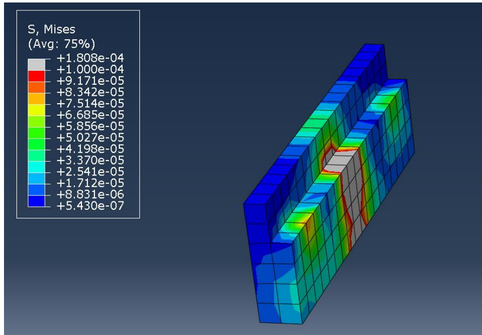
Ilustración 15 Modelo del estribo sin cargas de presión de agua MPa
