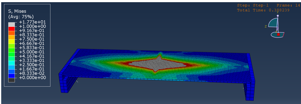
Ilustración 16 Modelo general analizado en FEM MPa
