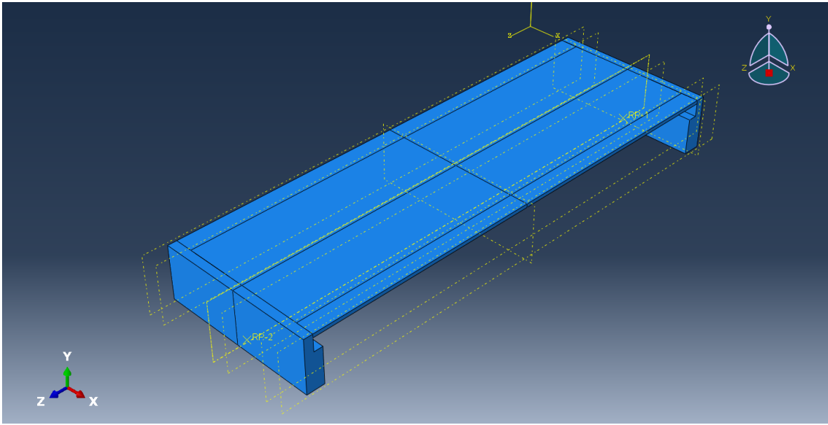
Ilustración 31 Ensamblaje del modelo
