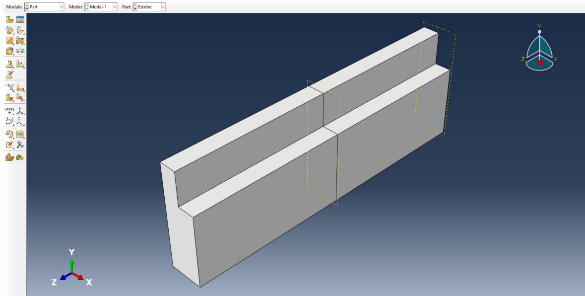
Ilustración 29 Creación de partes para análisis FEM
