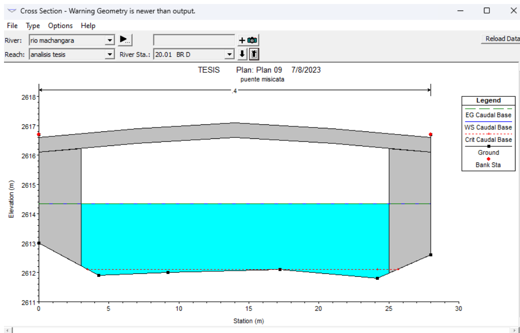
Ilustración 8 Modelo de puente en EL PROGRAMA DE ANÁLISIS DE CRECIDAS
