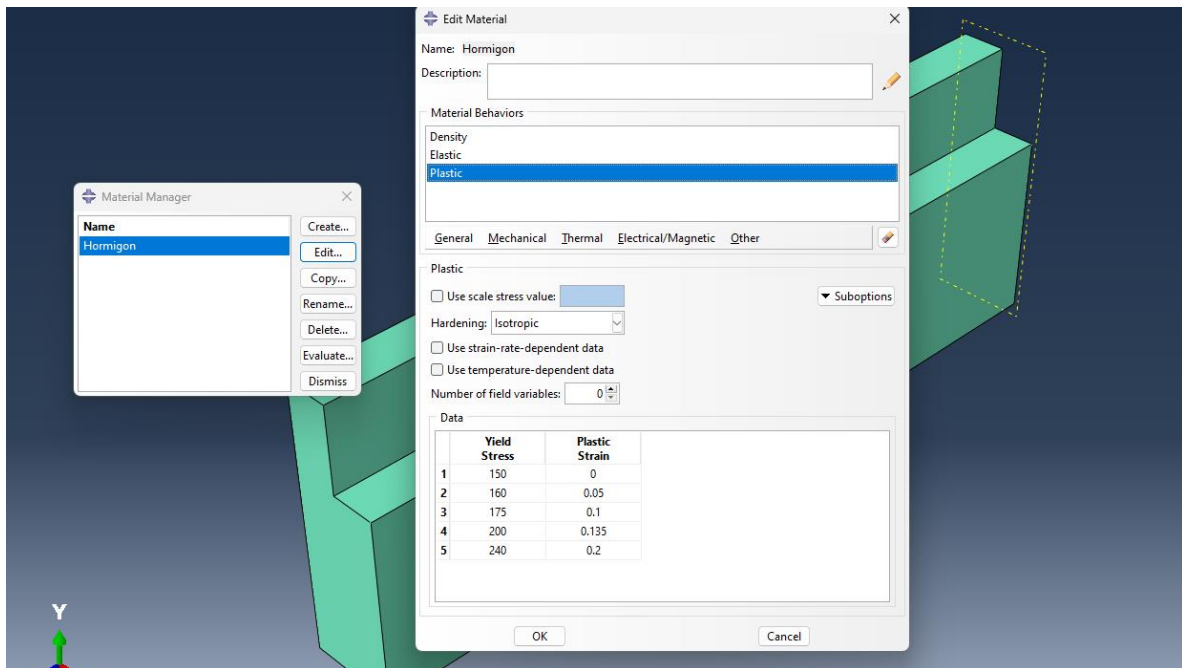
Ilustración 30 Propiedades del hormigón para el modelo
