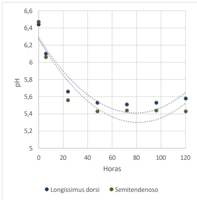
Figura 1. Variaciones Temporal del pH en relación al musculo.
