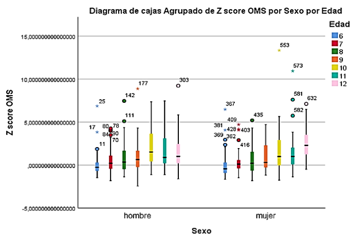
Figura 2. Diagrama de cajas agrupado
