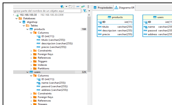
Figura 4. Diagrama de base de datos
