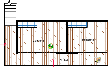
Planta Nivel: -3.06 Escala: 1:200
