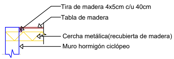
Detalle Constructivo 6 Escala: 1:0.25
