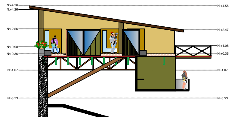
Corte G-G Escala: 1:200
