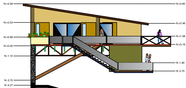
Elevación Lateral Izquierda Escala: 1:200
