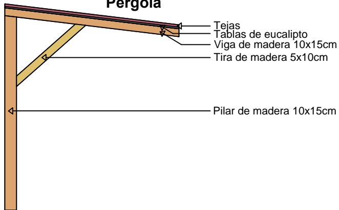
Detalle Constructivo 4 Escala: 1:50
