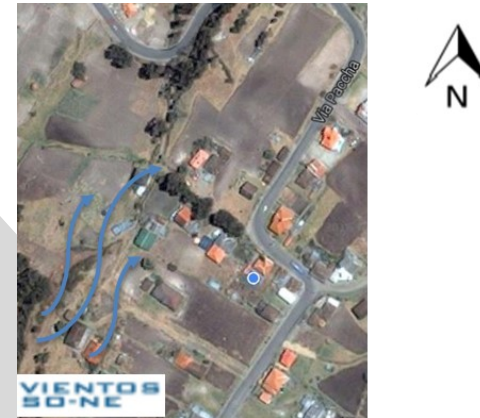
Ilustración N°16. Vientos predominantes
