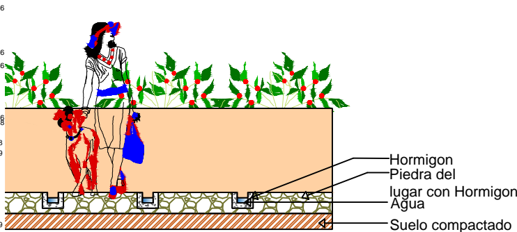
Detalle Constructivo 5 Escala: 1:50
