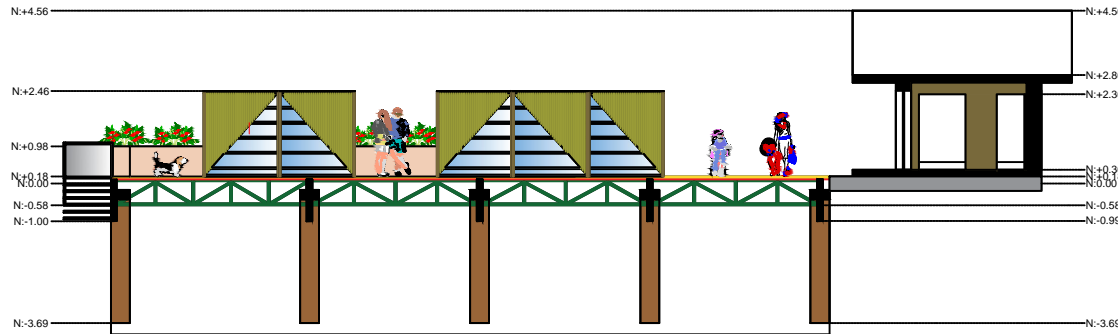
Corte F-F Escala: 1:200
